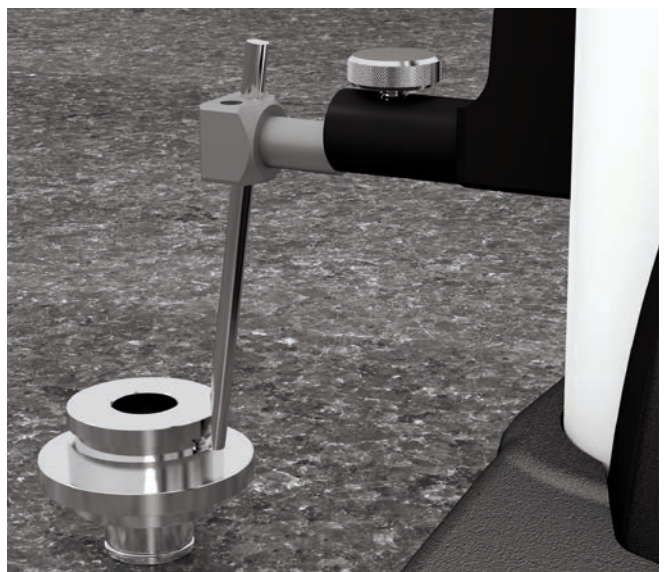
Determinazione dell'altezza di una scanalatura su un pezzo integrato in uno strumento di misura per l'endoscopia
